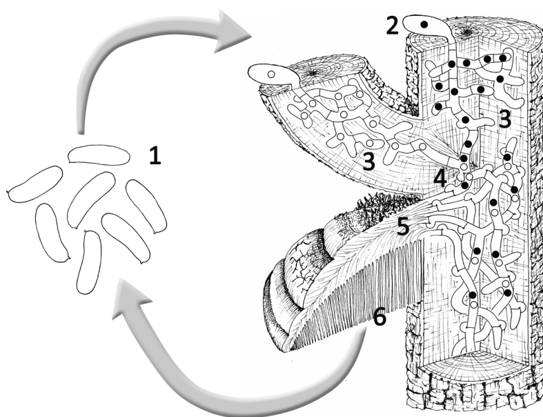
Figura 1. Ciclo biológico de un hongo la madera: 1, esporas microscópicas que se dispersan por el viento; 2, espora que se pone en contacto con la madera y germina; 3, desarrollo del micelio primario monocariótico dentro de la madera; 4, las hifas de micelios de distinta polaridad se conjugan y el nuevo micelio pasa a tener dos núcleos (micelio secundario dicariótico); 5, desarrollo del basidioma o cuerpo de fructificación, el micelio que lo constituye se denomina terciario; 6, en el himenóforo del basidioma se producen las esporas que serán dispersadas y colonizarán nuevos sustratos leñosos.
