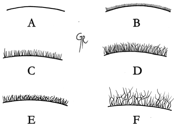
Figura 11: Diferentes texturas de la superficie del píleo: A, glabra; B, pubescente; C, velutinoso a hispido; D, viloso; E, tomentoso; F, hirsuta (Tomado de Robledo & Urcelay 2009).
